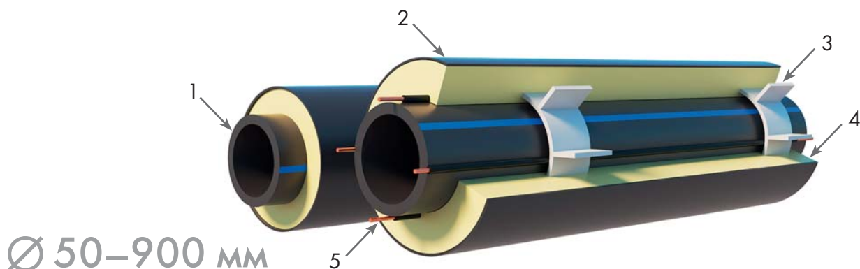
Труба АЛЬФА
