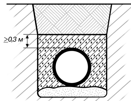
Рис. 4.3 Обсыпка трубопровода
