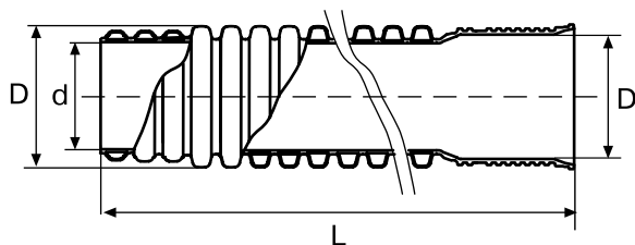
Труба ИКАПЛАСТ с раструбом исп. 2 (с уменьшенной высотой гофра в месте соединения с раструбом) Класс жесткости SN8
