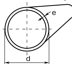
Размеры труб ИКАПЛАСТ из полиэтилена для газопроводов по ГОСТ Р 50838-2009
