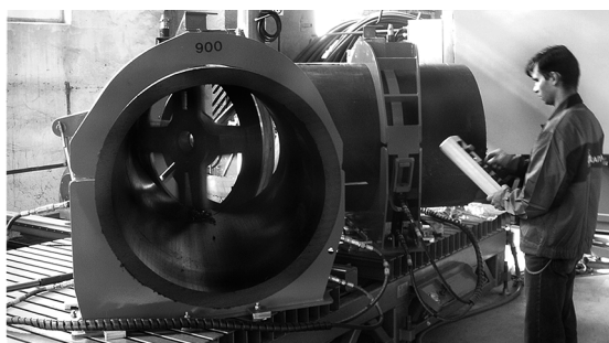
Фото 4.2.2. Производство соединительных деталей ИКАПЛАСТ в заводских условиях
