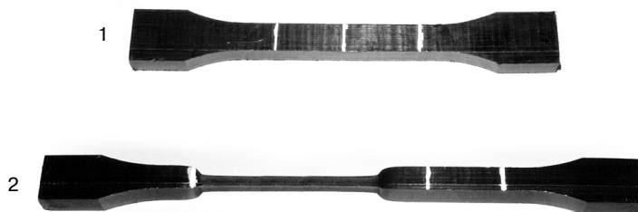
Фото 3.1. Испытание ПЭ трубы на осевое растяжение (относительное удлинение при разрыве) является одним из эффективных способов проверки качества труб при осуществлении входного контроля.
