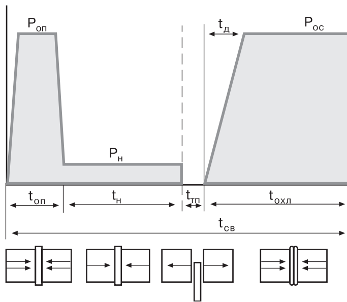
Рис. 4.2.13. Циклограмма сварочного процесса
