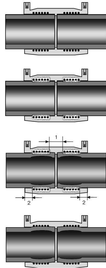
Рис. 4.2.5. Процесс сварки муфтой с ЗН
