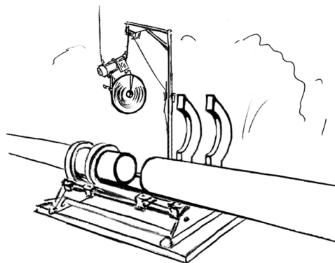
Рис. 4.2.6. Закрепление и центровка труб в зажимах центриатора сварочной машины
